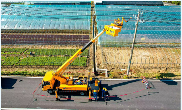
带电作业机器人进行带电搭接
